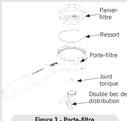
Figure 3 - Porte-filtre
